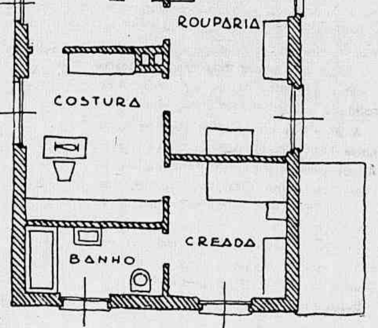
PLANTA DO 2º PAVTO ESCALA 1:100
