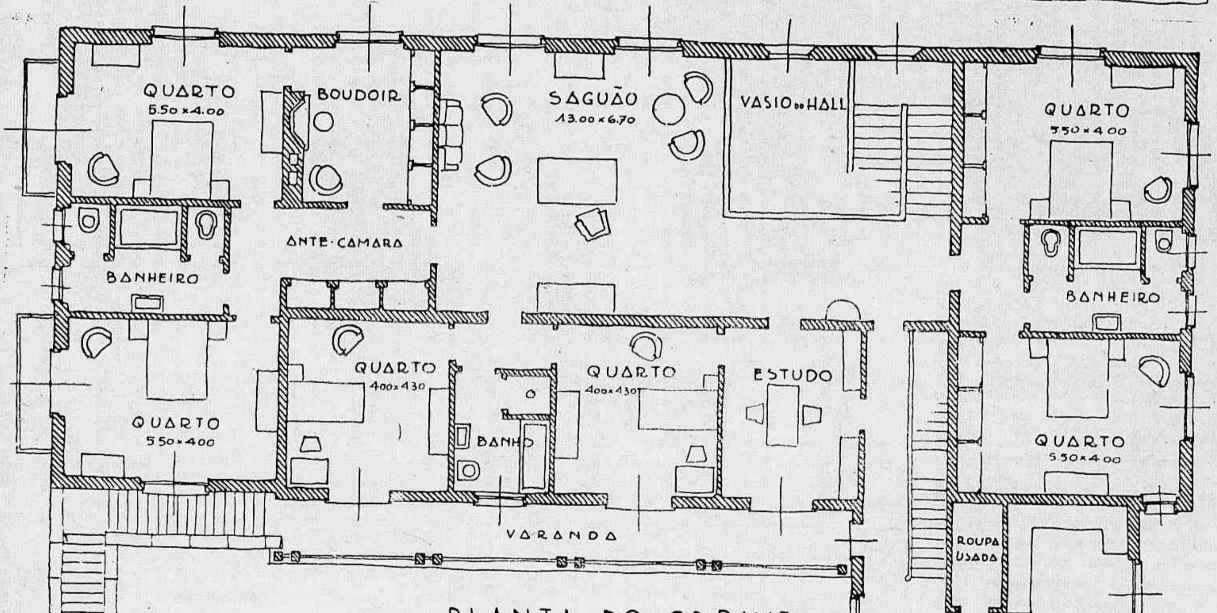
PLANTA DO 2º PAVTO ESCALA 1:100
