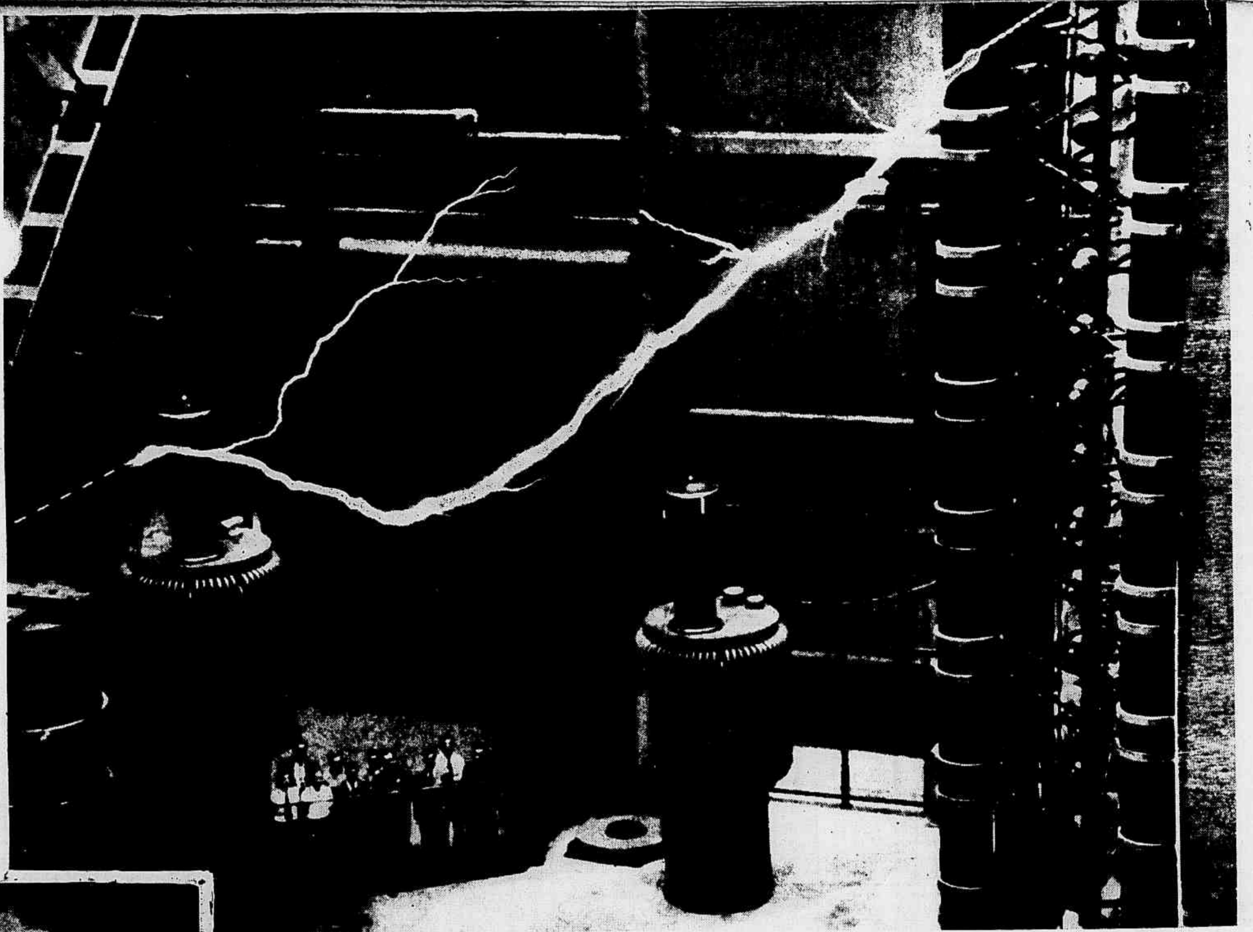
O MAIOR GERADOR de relâmpagos e trovões artificiais existente no mundo, com a força de 15 milhões de volts, fabricado pela General Electric, nos laboratórios de Pittsfield, Massachusetts. Ao lado, reprodução de gravura antiga, mostrando a cena histórica do papagaio de Benjamin Franklin, base do pára-raios.
