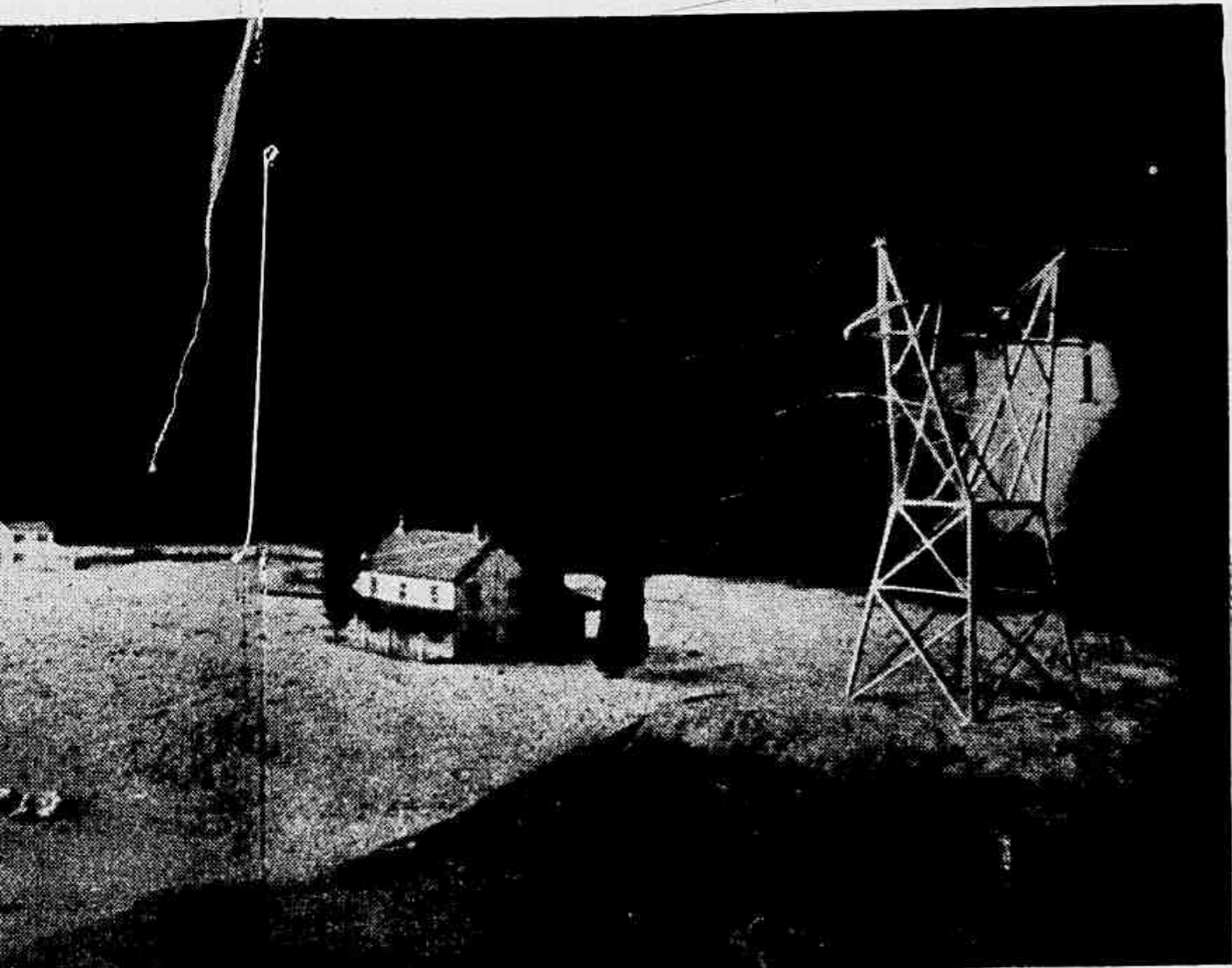
alvo da negativa, vinda das nuvens. Em baixo: outra experiência desta vez científica da Westinghouse numa aparelhagem de três milhões de volts, mostrando como defender as casas
