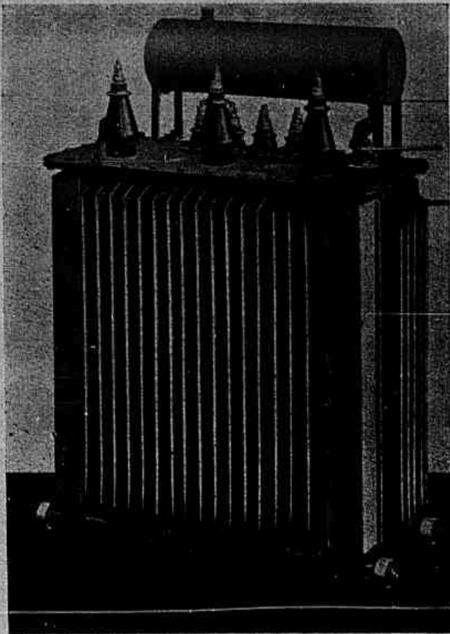
Transformadores até 600 KVA. Construídos no Rio e em S. Paulo.
