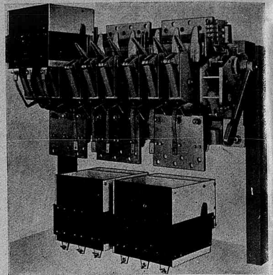
Chave automática a óleo, montada no país — 4.000 ampères
