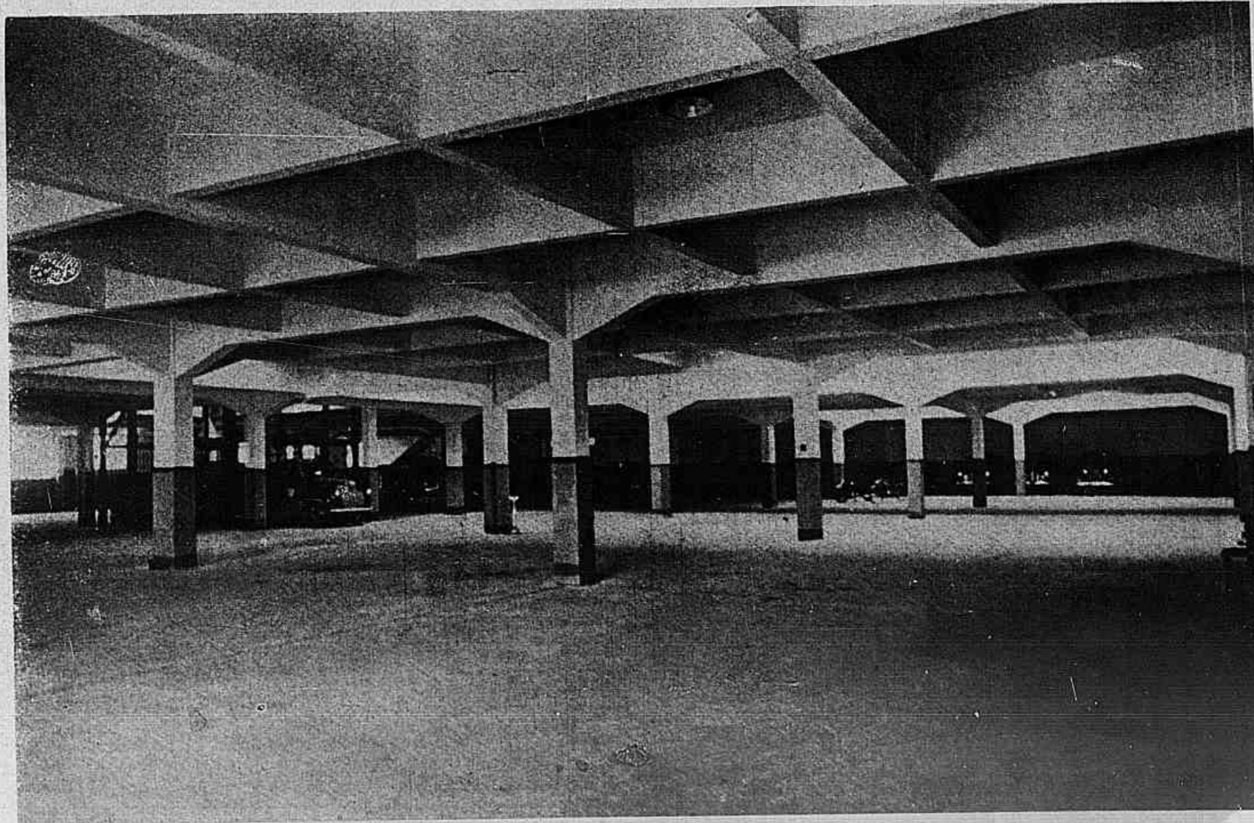
Garage do Serviço Rodoviário
