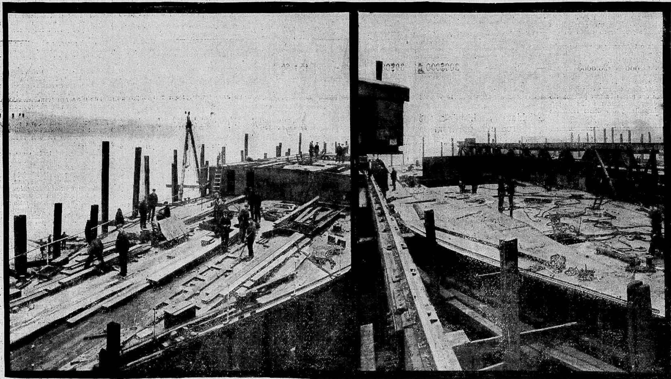
Monitores em construção para a nossa esquadra, na Inglaterra. As photographias mostram o adiantamento das obras
