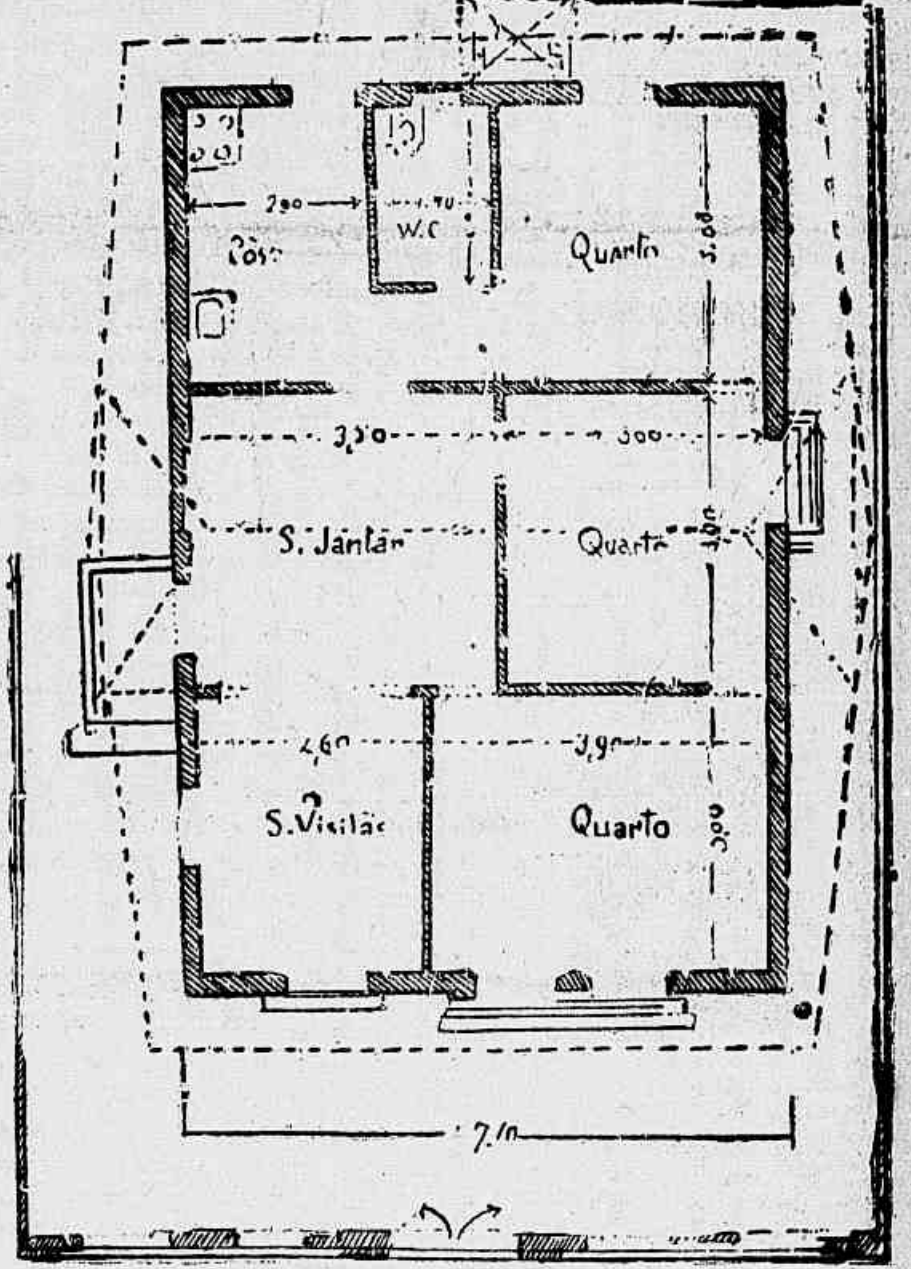
PLANTA HORIZONTAL
