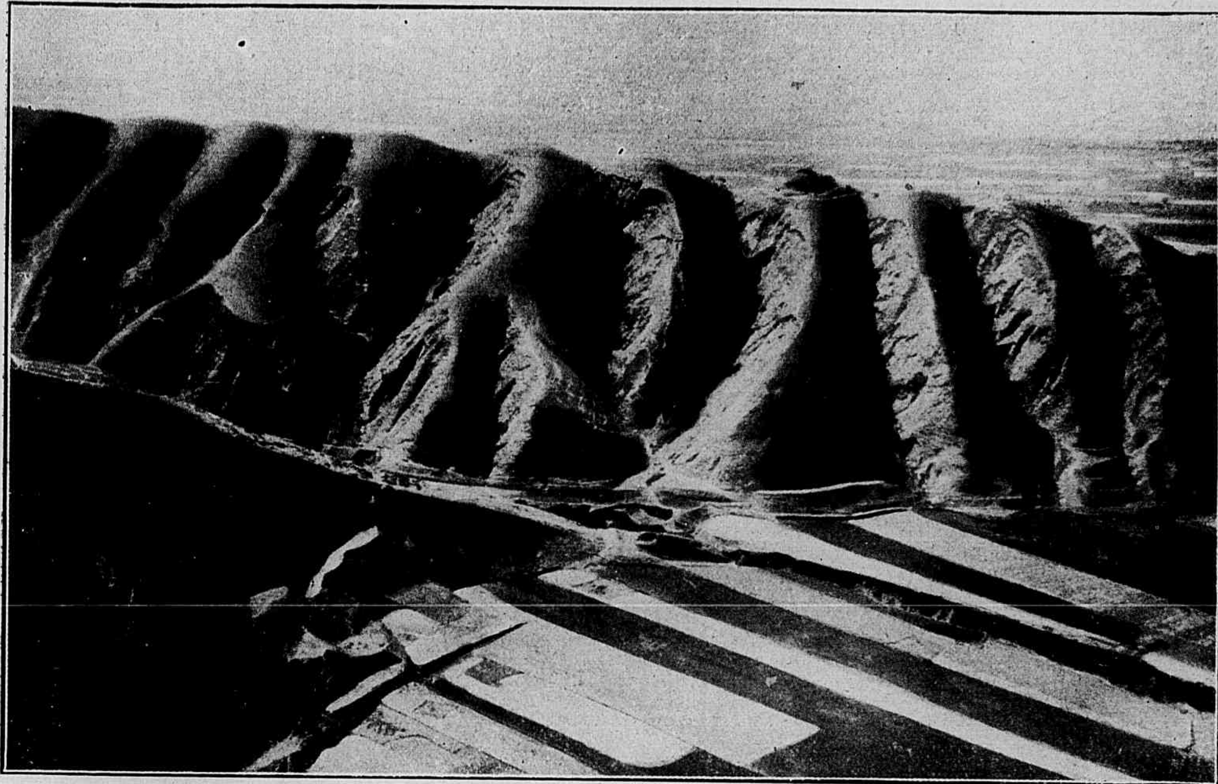
Parece um monstro ante-diluviano, imerso, com vertebrae bem salientes. É uma montanha calcarea, trabalhada pelas chuvas, na região de Lanhou.
