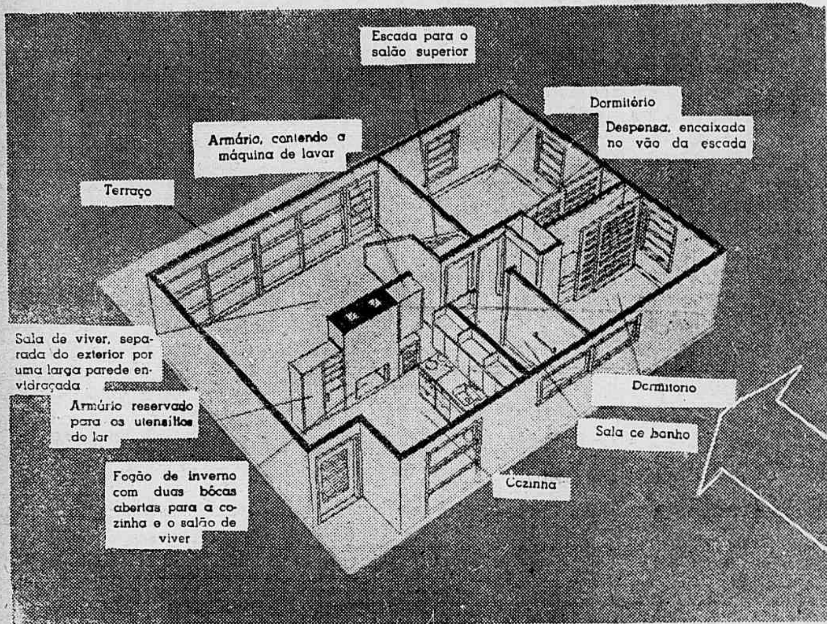
Eis a planta geral da casa pre-fabricada. Iguais a essa estão construindo quatro por hora, nos subúrbios de Nova York
