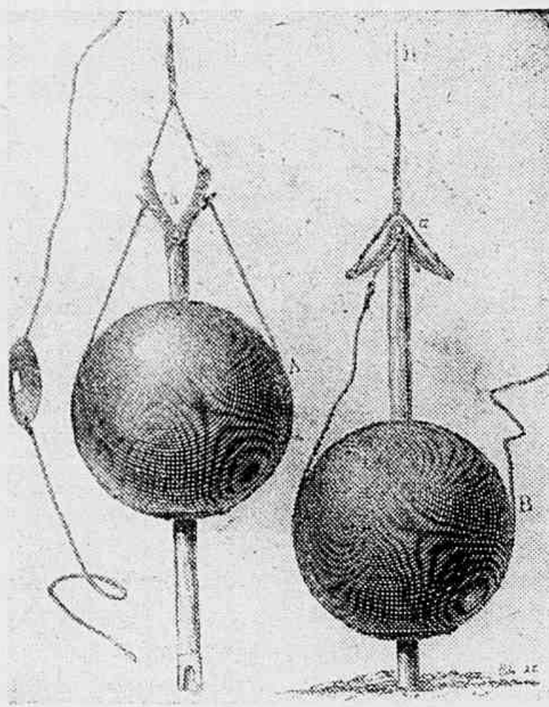
Sonda de Brooke para pesquisar as profundezas do mar
