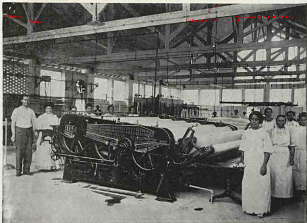
Uma machina que pesa 20 toneladas, destinada a passar a roupa lisa, — sete lençoes por minuto.
