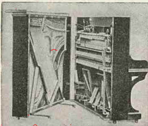
AUTO PIANO FECHADO AUTO PIANO ABERTO DE 65 E 88 NOTAS
