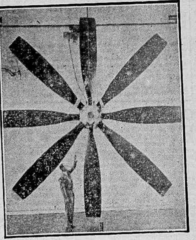
NOVO PROPULSOR DE AVIAO — A "Curtis-Wright Corporation" fabricou este propulsor de avião, denominado "Octoprop", por abreviatura, e que é considerado o maior do mundo. Dotado de 8 pás, o novo propulsor tem mais de 19 pés de diâmetro (cerca de 5,8 metros), assemelhando-se muito a um grande polvo. Destina-se a ser usado com turbo-motores de 10.000 e 15.000 H. P. (Foto ACME, para o JORNAL DE NOTÍCIAS)
