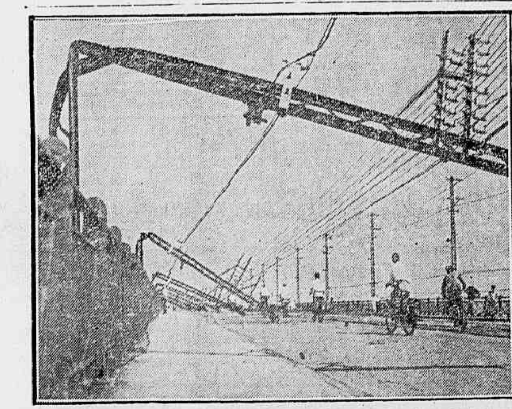
EFEITOS DE UM FURACÃO — A gravura mostra postes de aço retorcidos de forma idêntica por um tremendo furacão e interrompendo o trajeto num dos lados da ponte de Yodo, em Osaka, no Japão. Esse furacão, que foi dos mais violentos desta última década, causou grandes estragos na zona Kobe-Osaka. Mais de 100 pessoas foram mortas e cerca de 1.000 ficaram feridas. (Foto I. N. S., para o JORNAL DE NOTÍCIAS)
