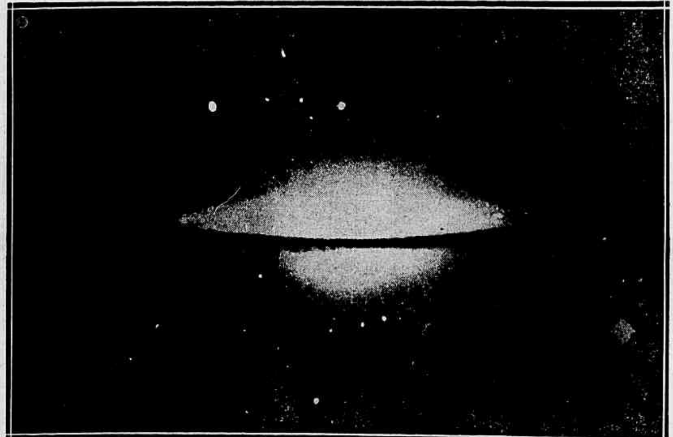
A nebulosa "Messier cento e quatro", fotografada pelo telescópio do Mt. Palomar; distando vários milhões de anos-luz, pode dar uma nitida ideia da grandiosidade da criação, somente revelada ao espírito humano pela luz da Astronomia
