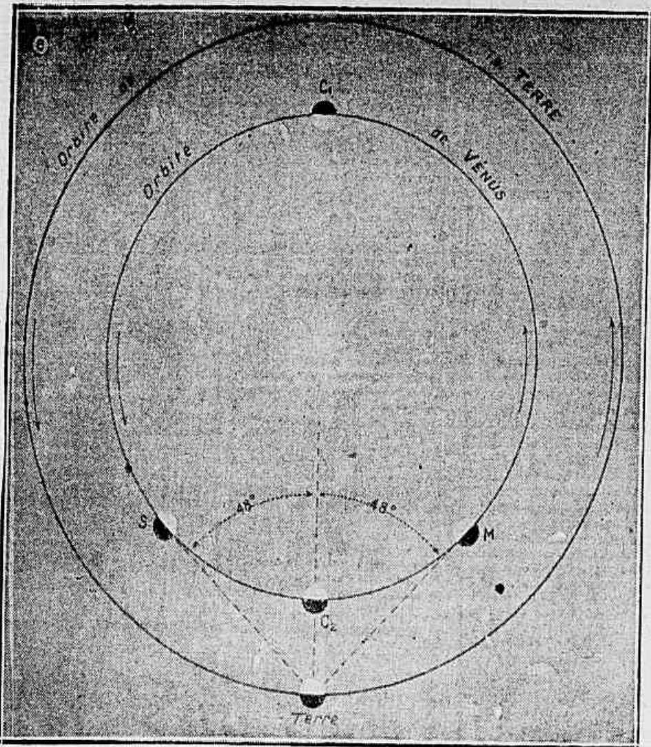
Foi a astronomia que nos revelou as leis que regem os corpos celestes; graças a elas, os fenômenos que periodicamente ocorrem podem ser previstos com grande antecipação.
