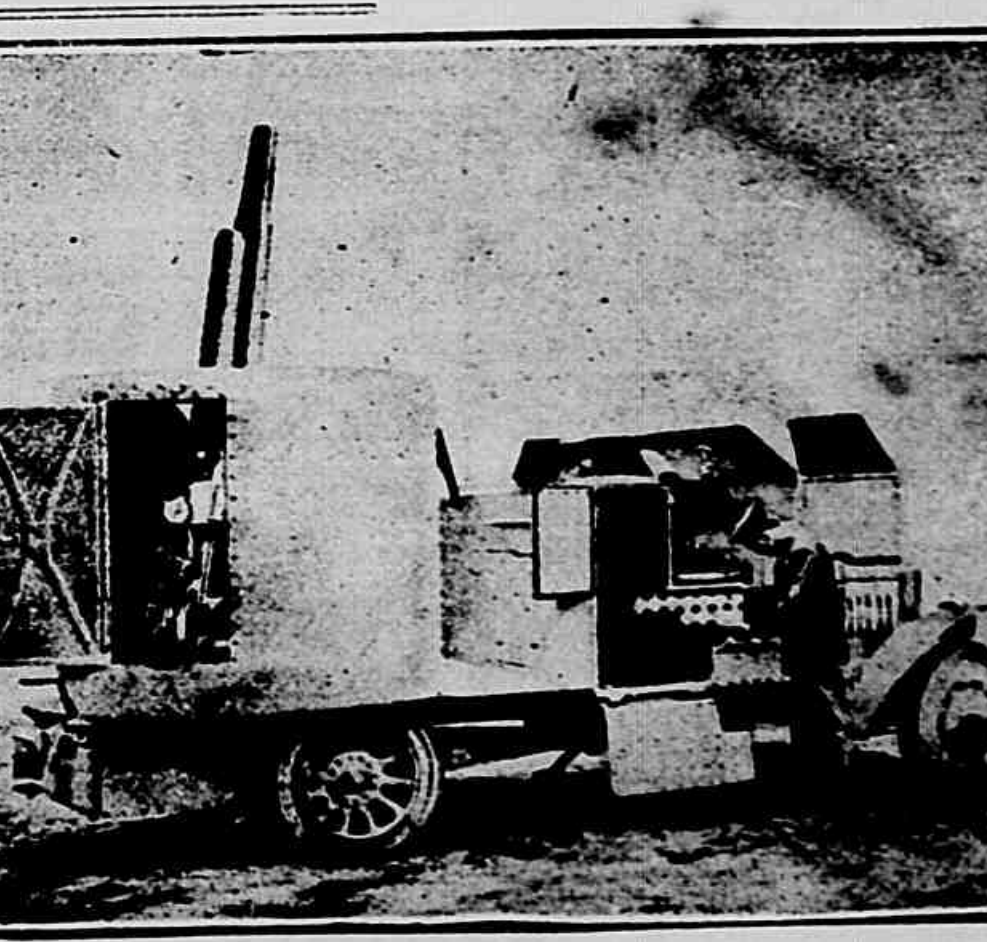
Canhão do exercito allemão, de 71 milímetros, contra aeroplanos, montado em um automovel blindado
